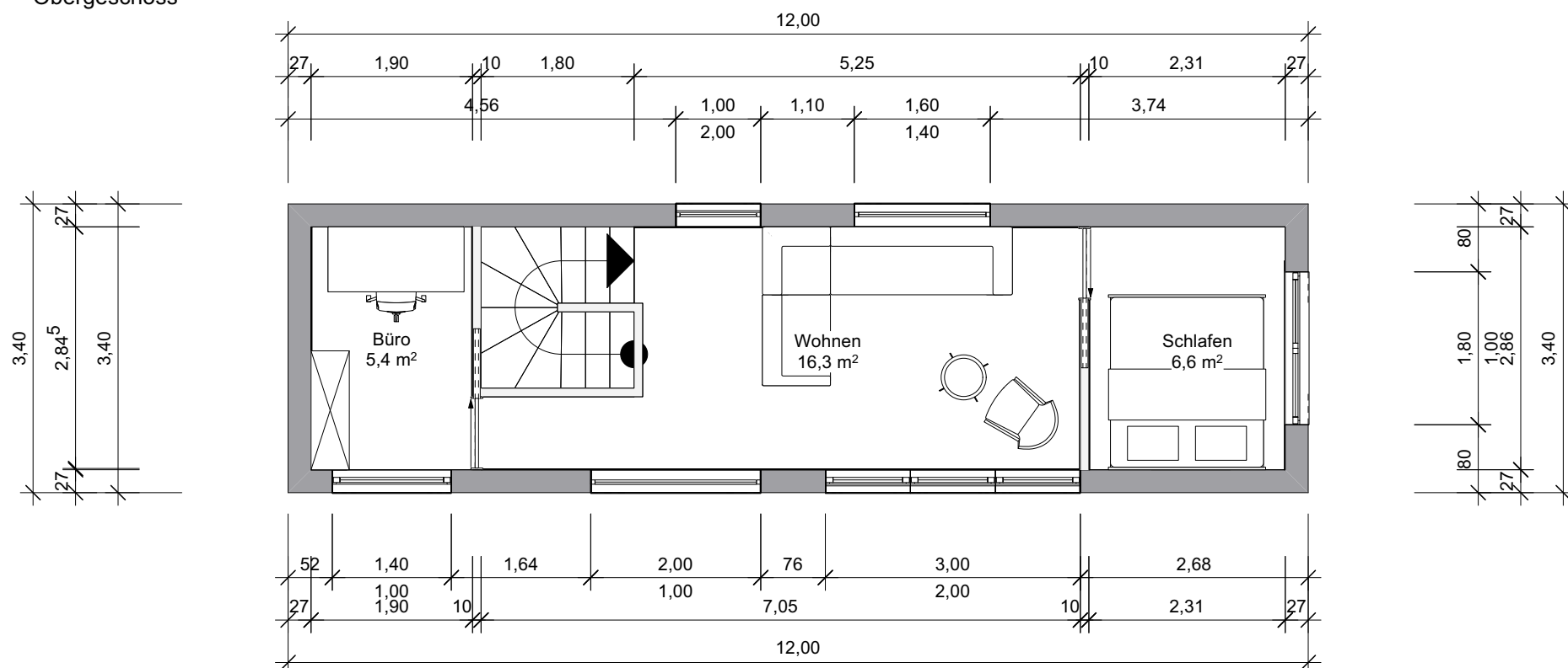
Grundriss Obergeschoss
